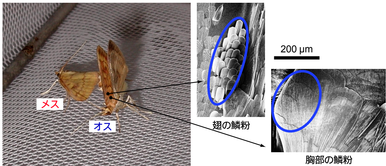
図1a: アワノメイガの発音行動と発音器官。オスは交尾の前に翅と胸部にある特殊な鱗粉を摩擦させて超音波を出します(動画1、動画2も参照)。
