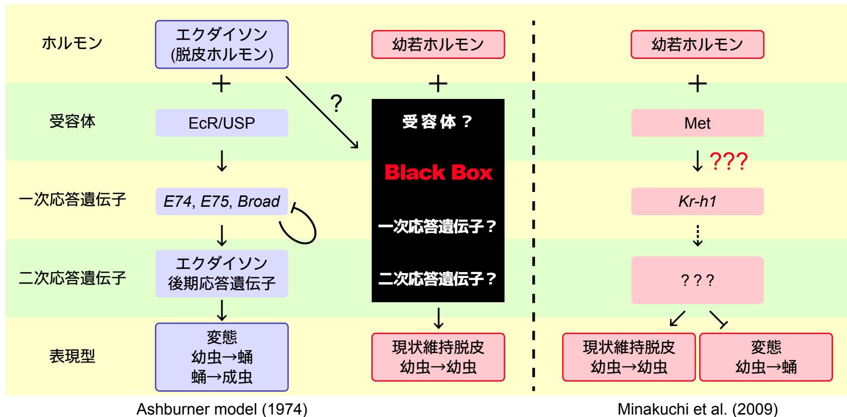
図2: 幼若ホルモンと脱皮ホルモンの分子機構
