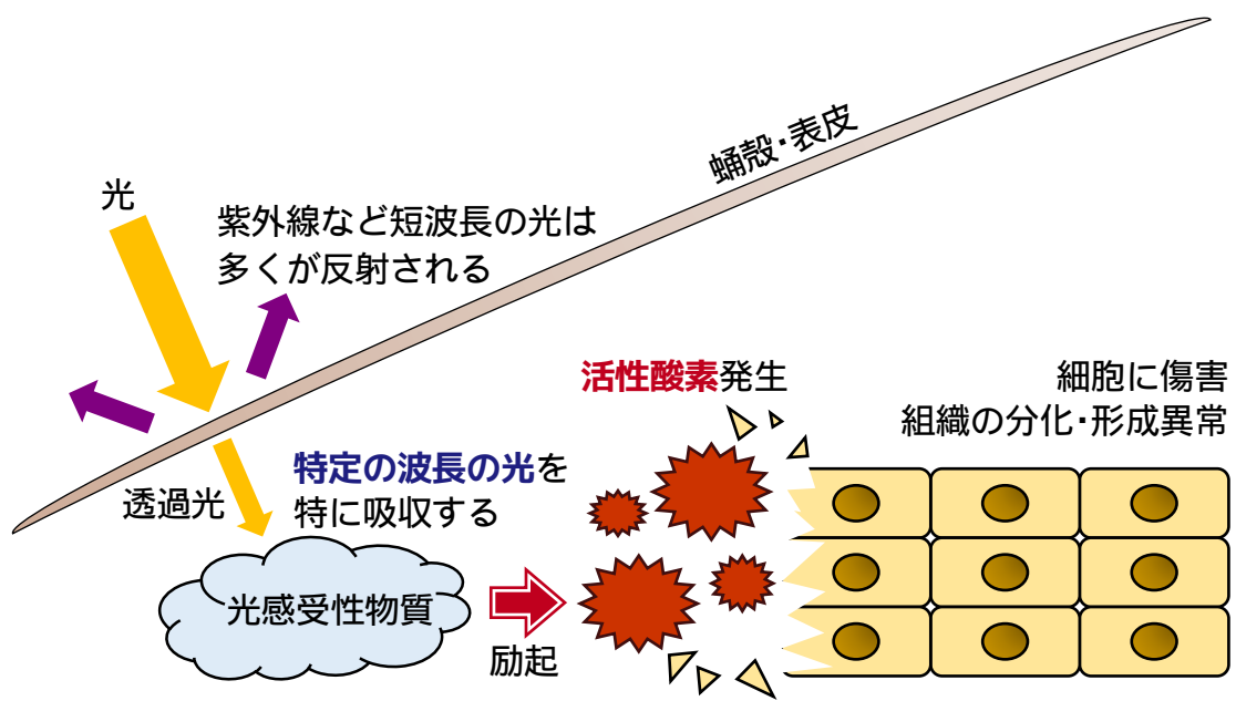
図3: 予想される殺虫メカニズムの模式図。青い光の照射によって活性酸素が発生し、組織や細胞がダメージを受ける可能性がある。
