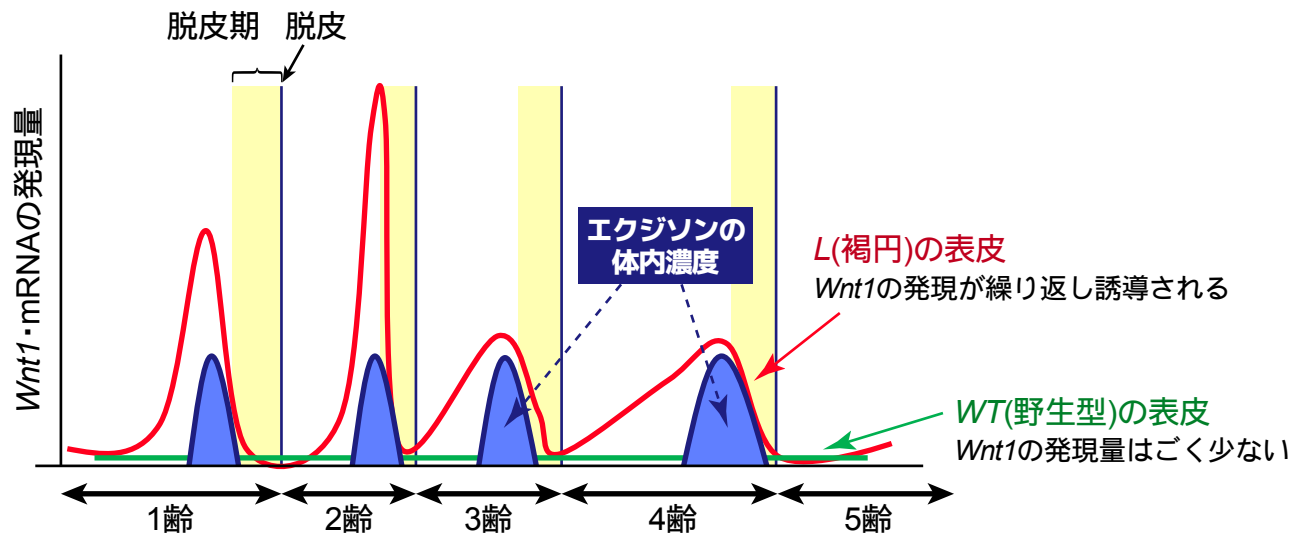
図2: カイコ褐円変異体(L)はWnt1の変異によって生じた。褐円の表皮では、Wnt1の発現が脱皮ホルモン(エクジソン)によって繰り返し誘導される。
